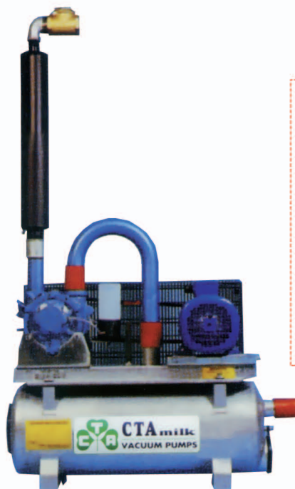
MZ-00-0001 (Καρβουνάκι) Αρμεκτική σε καζάνι 25lit. και κινητήρα 0,55Kw Παροχή 170 - 200lit./min Κατασκευή: Τουρκία ΤΙΜΗ - 550,00 €
